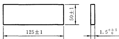
图2 试验板示意图
